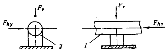
Схема нагрузок на опору 1 — труба; 2 — подвижная опора трубы
